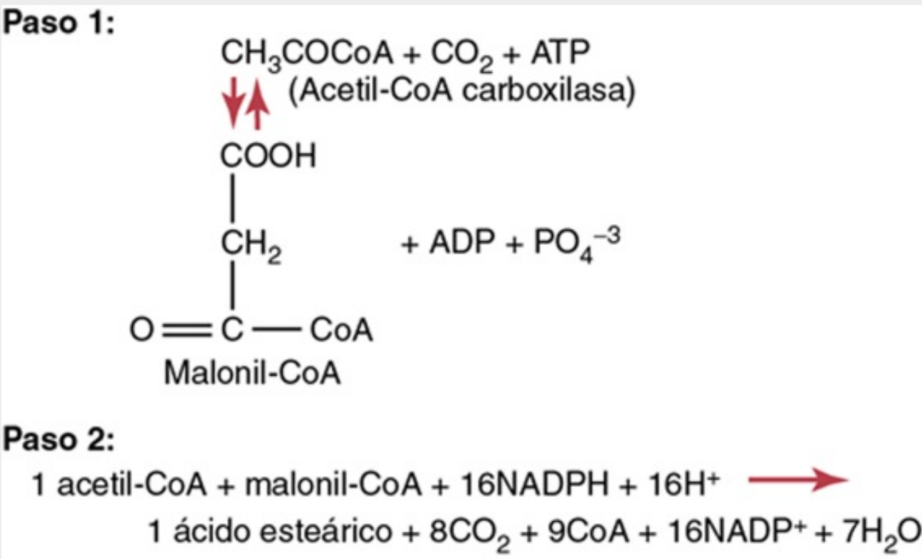
FIGURA 69-3 Síntesis de ácidos grasos.
